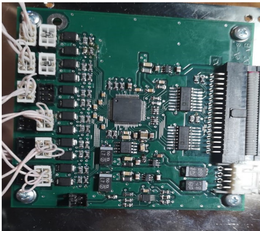
Рисунок 3: Плата АЦП. Каналы 0-2 (нижние) подключены без делителей. Канал 3 с базовым делителем. Каналы 4,5 с заглушками.
