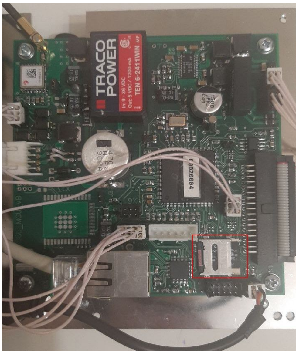
Рисунок 4: Процессорная плата регистратора. Красным обведён сокет SD-карты.
