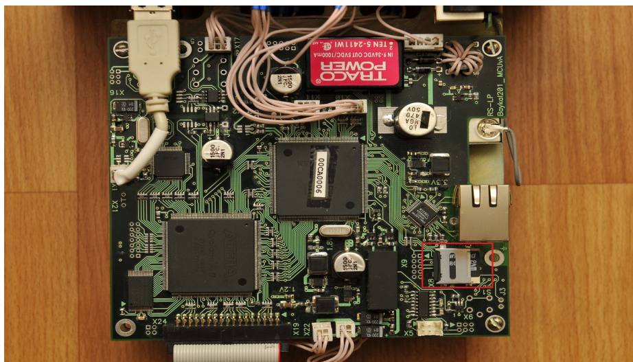
Рисунок 3: Процессорная плата регистратора. Красным обведён сокет SD-карты.
