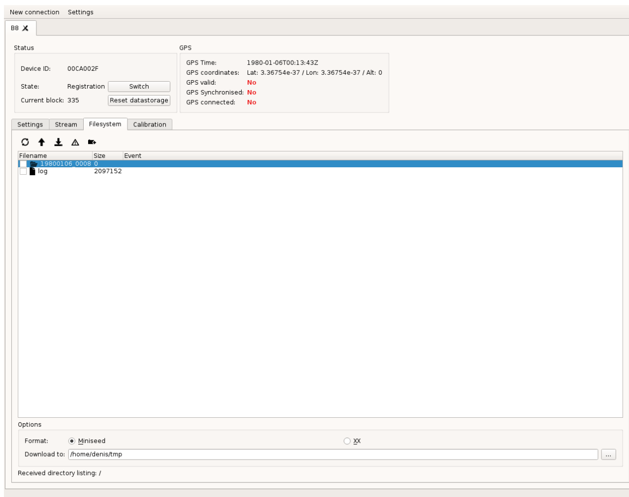
Рисунок 11: Вкладка Filesystem
