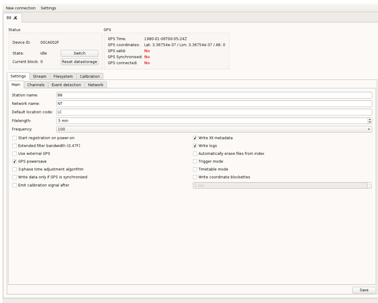
Рисунок 5: Вкладка Settings/Main
